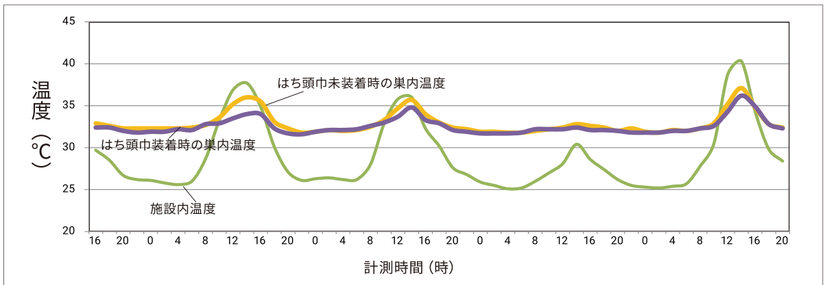
図 アグリ・トップクロマルキューブに、はち頭巾 (小) を装着した場合の温度推移 自社試験期間：2018年8月9日～8月13日
