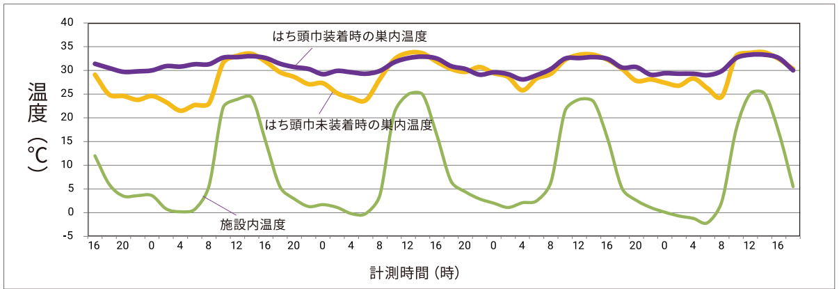
図 アグリ・トップクロマルキューブに、はち頭巾 (小) を装着した場合の温度推移 自社試験期間：2019年1月18日～1月22日
